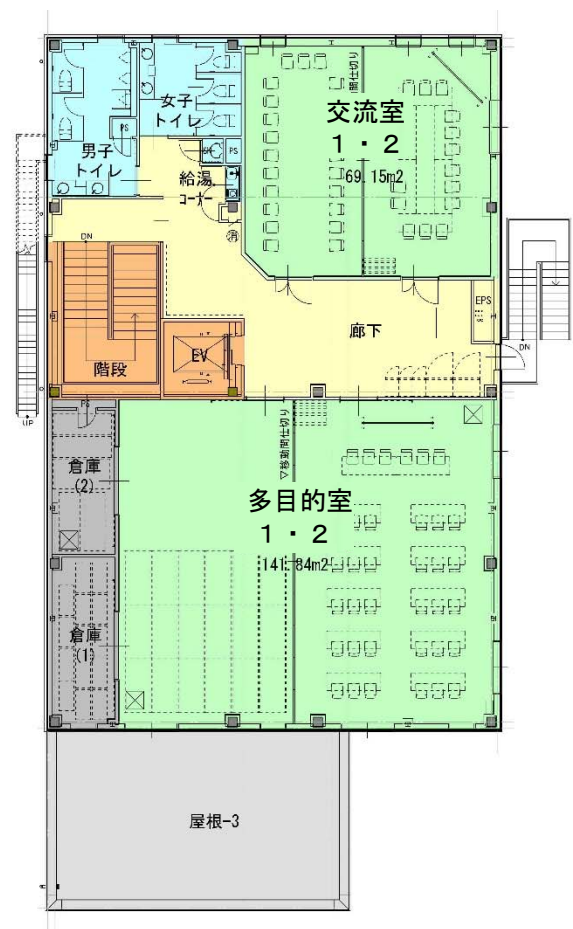
2 階平面図
