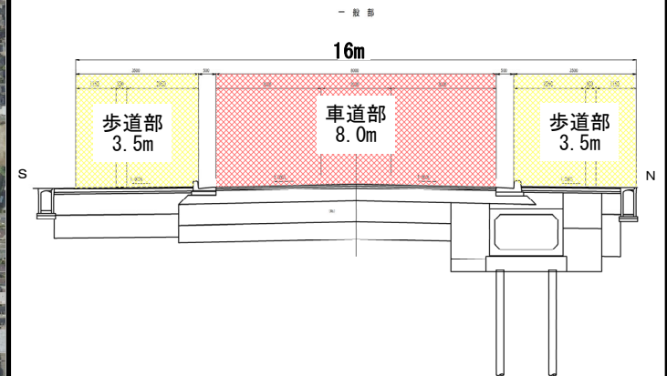
標準計画横断面図
