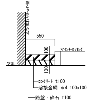
新設コンクリート部詳細図 S=1/30
