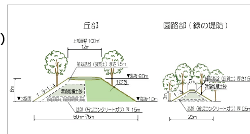
▲「千年希望の丘」第1号（構造図）
