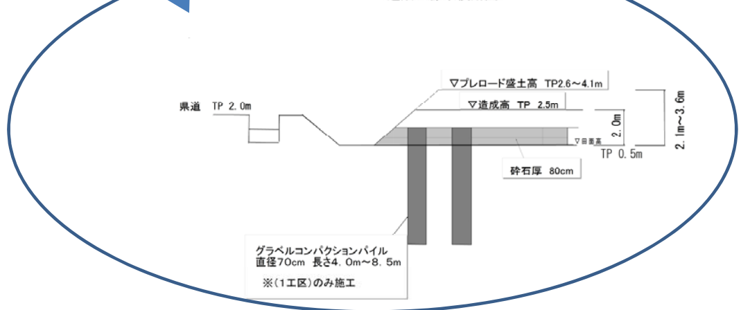
造成工標準横断面図
