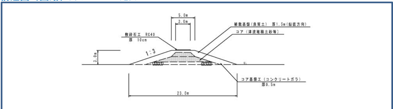
構造図（園路）高さ：3 m 延長：300 m
